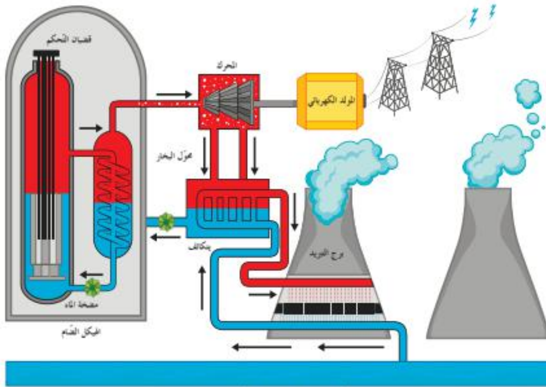
مراحل توليد الحرارة من الطاقة النووية
