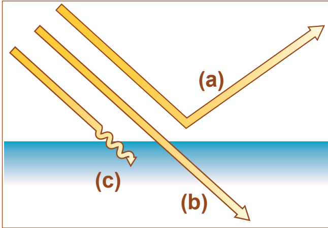
الشكل 10-3 الطرائق التي يتفاعل الضوء بها مع السطح. يمكنه أن ينعكس (a)، أو يخرق (b)، أو يتم امتصاصه (c).
