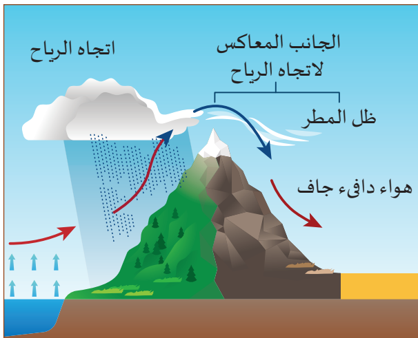
الشكل 19-3 تشكّل السلسلة الجبلية مناخين فرعيين.
