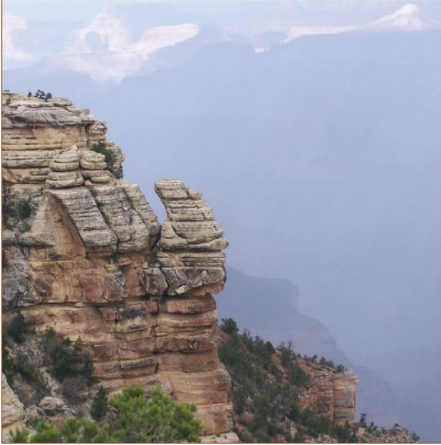
الشكل 1-2 تكشف صخري عند أعلى الأخدود.
