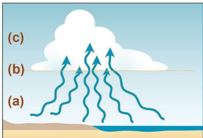
الشكل 29-1 مخطط لتكوّن الغيوم وصورة للغيوم: (a) يرتفع الهواء الرطب الدافئ، (b) الوصول إلى نقطة الندى، (c) تشكّل الغيوم.
