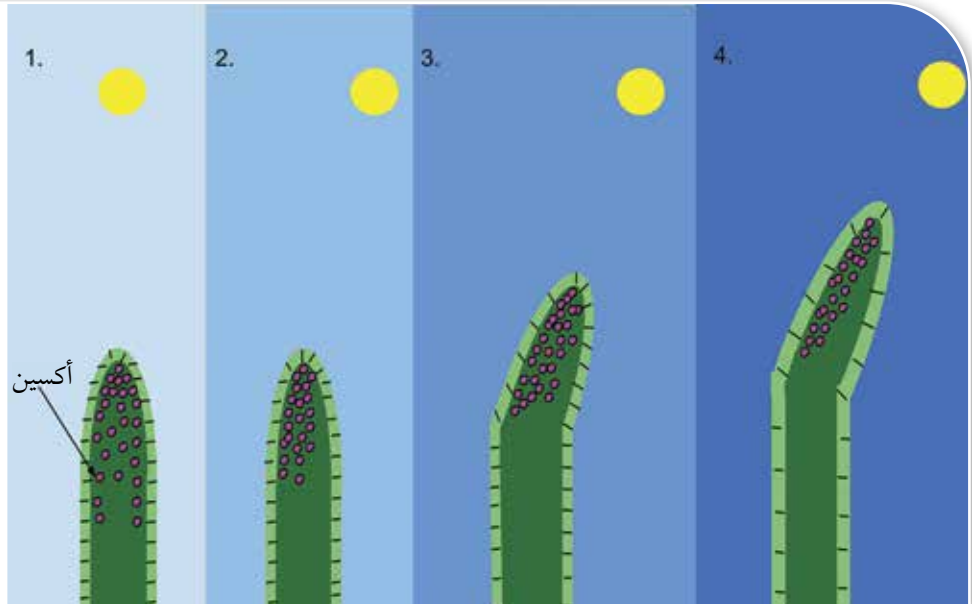
الشكل (14): انحناء البادرة في اتجاه الضوء.
