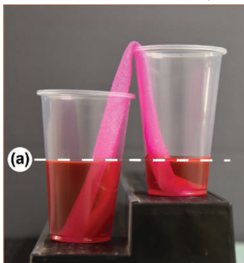
الشكل 3-47 كوبان موصولان بوسيلة الخاصيّة الشعريّة.
