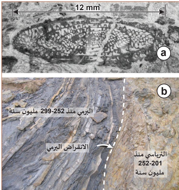
الشكل 19-2 (a) أحفورة بارافوسولينا، (b) الحدّ الفاصل بين البرمي والتراسي.
