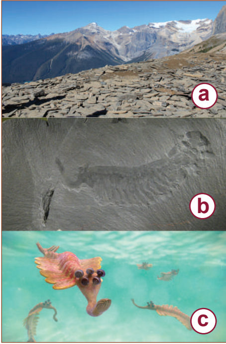
الشكل 14-2 (a) طين بورغيس الصفيحي، (b) أحفورة أوبابينيا، (c) رسم فنان للأوبابينيا.
