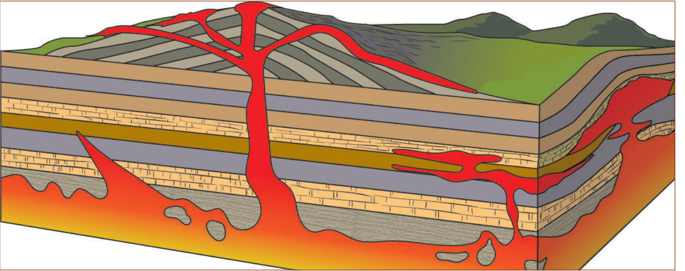
الشكل 2-26 رسم تخطيطي للاندفاعات النارية ضمن الطبقات الرسوبية.
