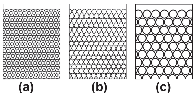
الشكل 10-3 لأحجام الحبيبات الثلاثة هذه المسامية نفسها تقريباً.
