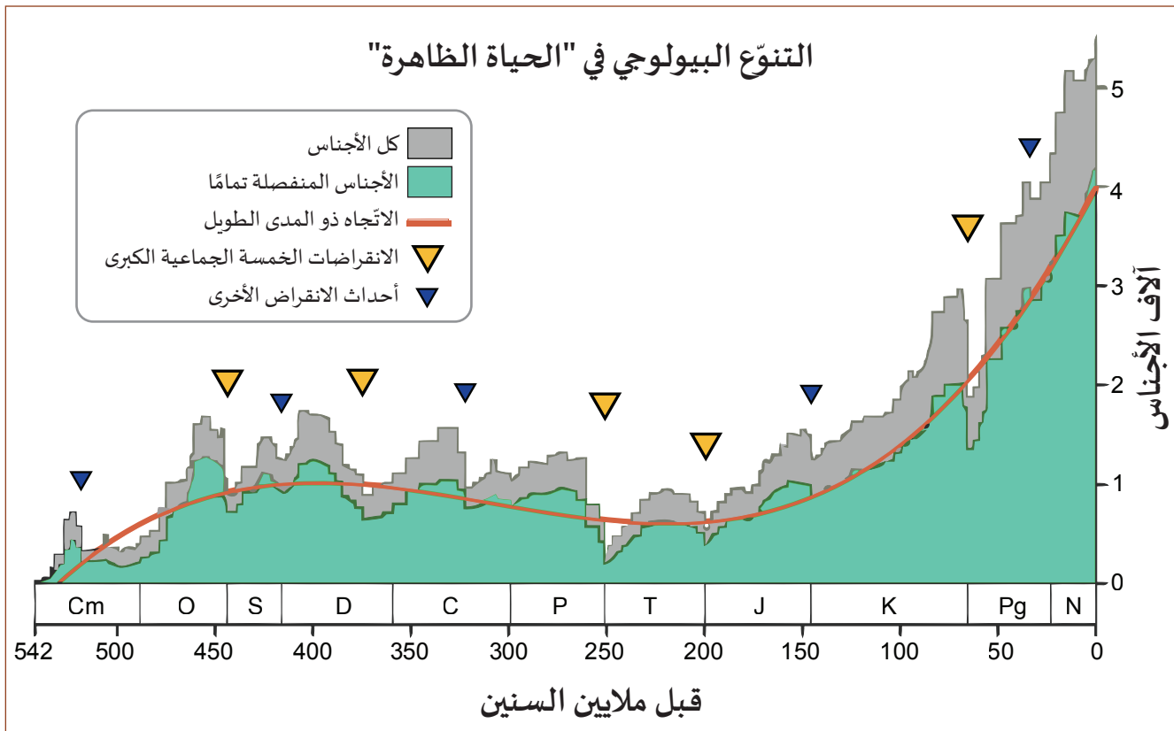
الشكل 7-2 مخطّط التنوّع البيولوجي وتأثير أحداث الانقراض.
