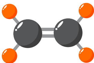
الشكل (2): الألكين متماثل.
