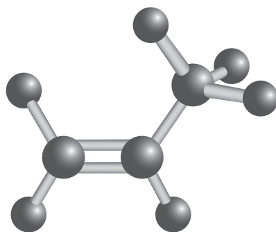
الشكل (3): الألكين غير متماثل.
