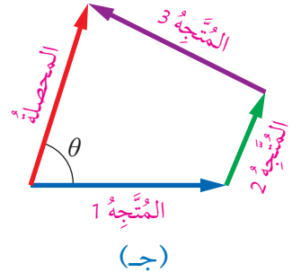
الشكل (17): محصلة مُتَّجِهَاتٍ عِدَّةً بطريقة المضلع.
