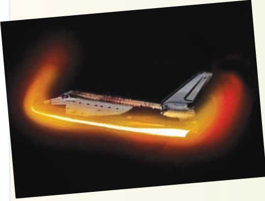
الشكل (١٥-٦): احتكاك جسم الموك بالغلّاف الجويّ.
