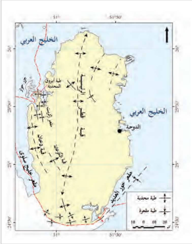
شكل (4) التركيب الجيولوجي لدولة قطر
