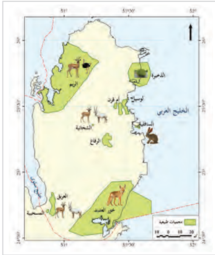
شكل (5) المحميات الطبيعية بدولة قطر
