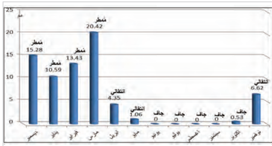
شكل (4) المعدّل الشهري لكمية المطر (مم) وحالة الشهور بدولة قطر من 1980 م - 2014 م
