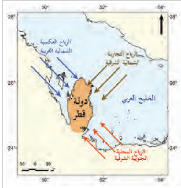
شكل (3) الرياح في قطر
