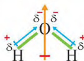
الشكل (31): العزم القطبي لجزيء H_2O .
