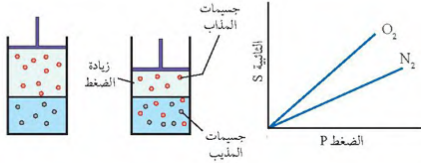
الشكل (7): العلاقة بين ذائبيّة الغاز وضغطه.
