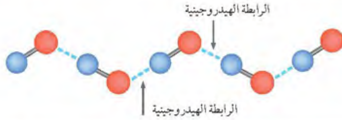
الشكل (32): الروابط الهيدروجينية بين جزيئات فلوريد الهيدروجين.
