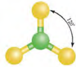
الشكل (25): الشكل الفراغي لجزيء BF_3 .
