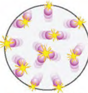
الشكل (3): التصادمات المرنة لجسيمات الغاز.
