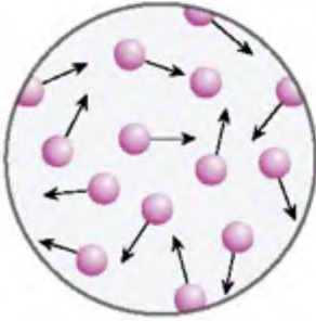
الشكل (2): الحركة العشوائية لجسيمات الغاز.
