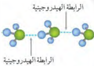
الشكل (33): الروابط الهيدروجينية بين جزيئات الأمونيا.
