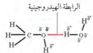
الشكل (35): الرابطة الهيدروجينية بين جزيئات الماء والميثانول.
