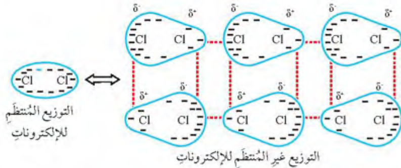
الشكل (38): تكوين قوى ثنائية القطب اللحظية بين جزيئات الكلور \text{Cl}_2 .
