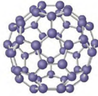
الشكل (23): جُزْيَةٌ واحدٌ من كُرّات باكي C_{60} .
