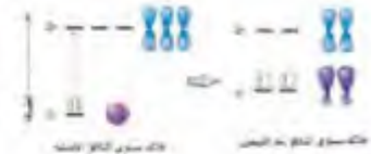
الشكل (27): توزيع الإلكترونات في أفلاك ذرة البيريليوم قبل التهجين وبعده.
