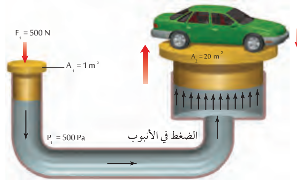
الشكل (10) المكبس المستخدم في رفع السيارات.
