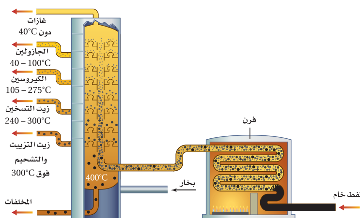
الشكل (4) برج التقطير التجزيئي للنفط موضحاً فيه درجات الغليان لمكونات النفط
