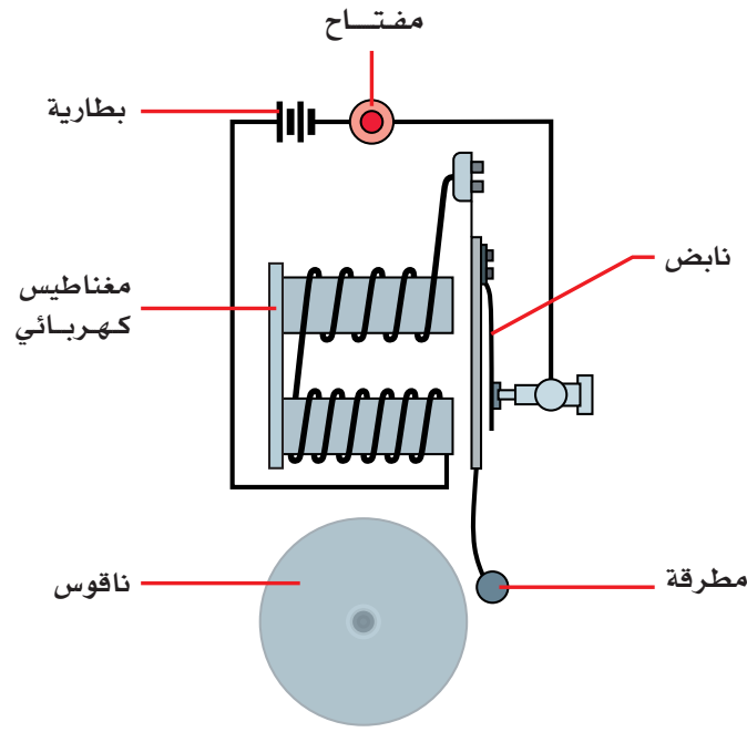
الشكل (9) آلية عمل الجرس الكهربائي
