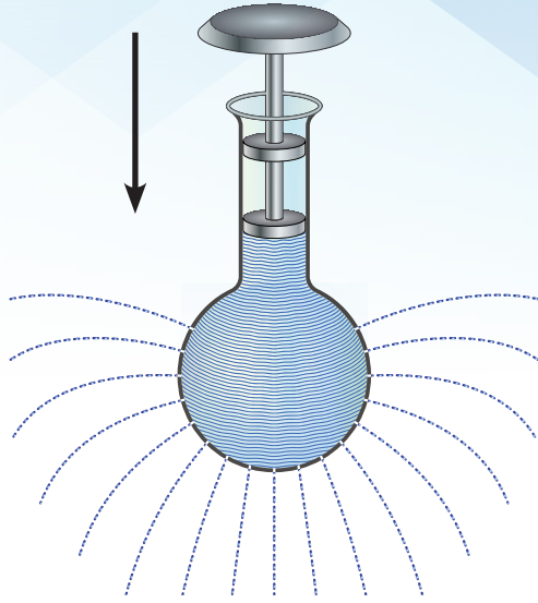
الشكل (8): تطبيق مبدأ باسكال
