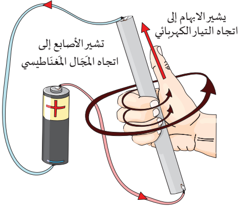
الشكل (4) تحديد اتجاه المَجَالِ المَغْنَطِيسِي حول سلك مستقيم.
