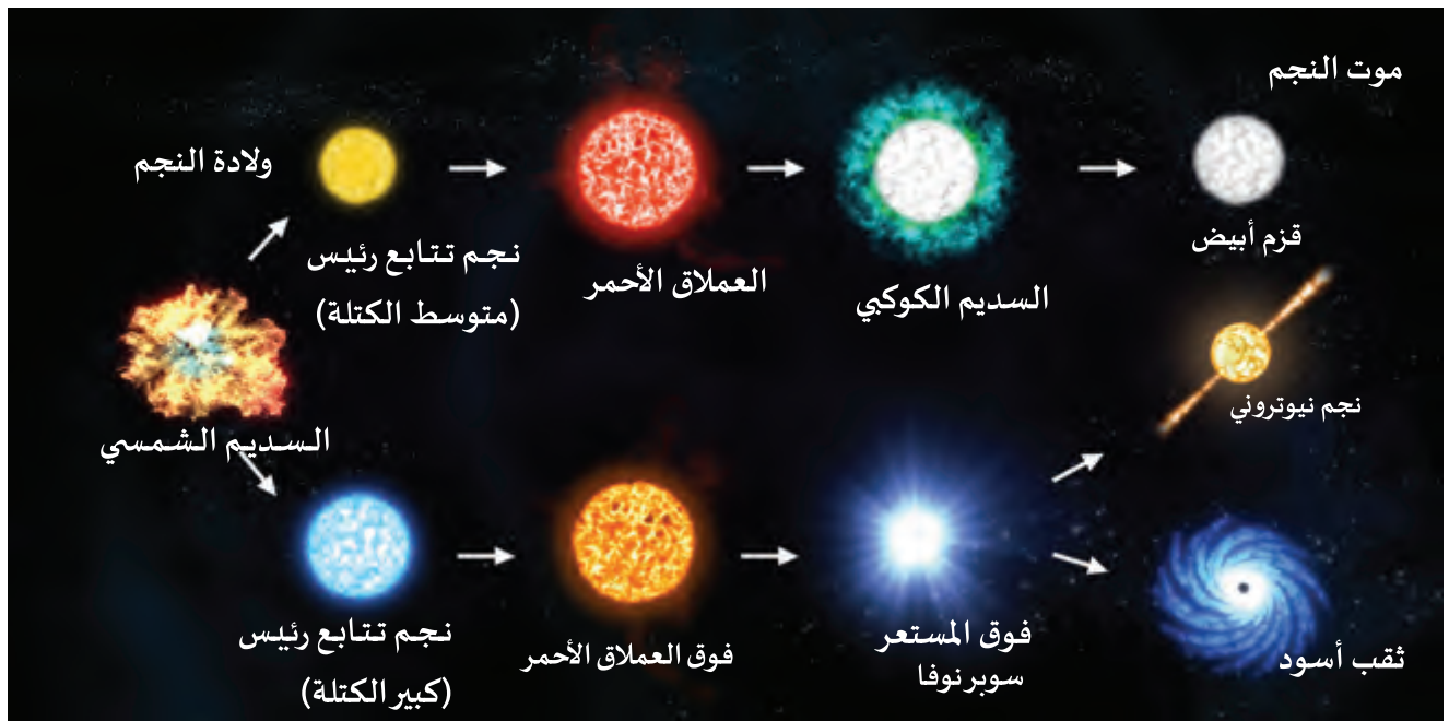
شكل (11): مراحل دورة حياة النجوم الصغيرة والكبيرة.
