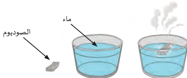
الشكل (1) تفاعل الصُّوديوم مع الماء
