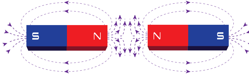
الشكل (3b) خطوط المجال المغناطيسي لمغناطيسين في حالة تنافر
