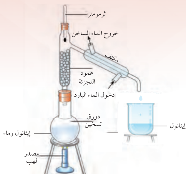
الشكل (3) جهاز التقطير التجزيئي
