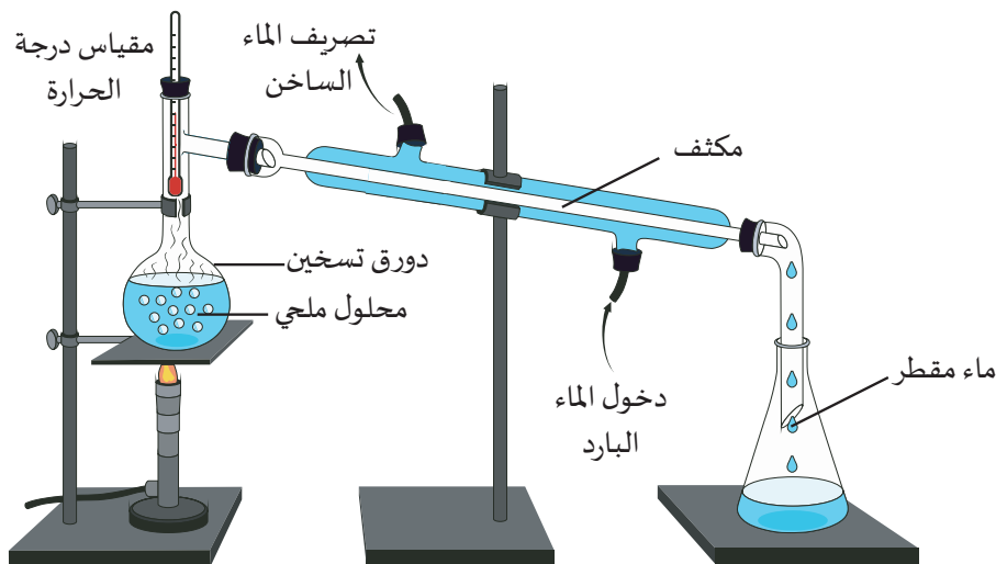
الشكل (2) جهاز التقطير البسيط
