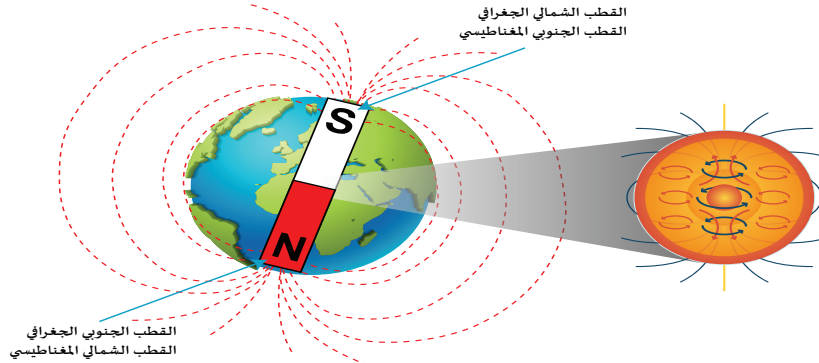
الشكل (4) خطوط المَجَال المغنطيسي للأرض
