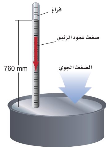
الشكل (5) تجربة تورشلي لقياس الضغط الجوي عند مستوى سطح البحر
