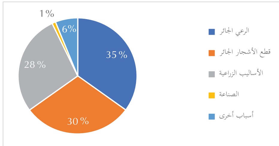
شكل (2) أسباب تدهور التربة.
