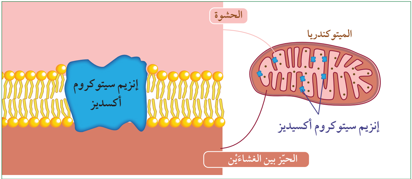
الشكل 22-3 إنزيم CcOX جزء من المسار الكيميائي الذي ينتج ATP في الميتوكوندريا.
