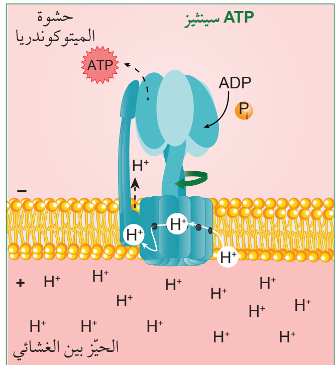
الشكل 26-4 يستخدم ATP سينثيز المنحدر الكهروكيميائي ليخزن الطاقة الكيميائيّة في روابط الفوسفات.
