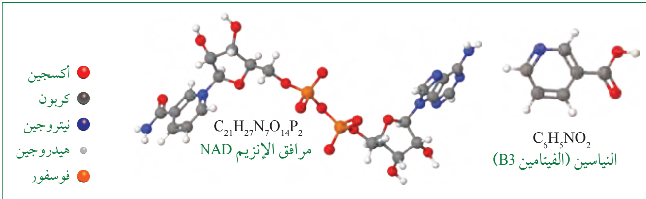
الشكل 23-3 الفيامين B3 ومرافق الإنزيم NAD.
