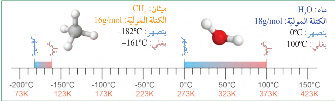
شكل 9-1 مقارنة درجات انصهار وغليان الماء والميثان.
