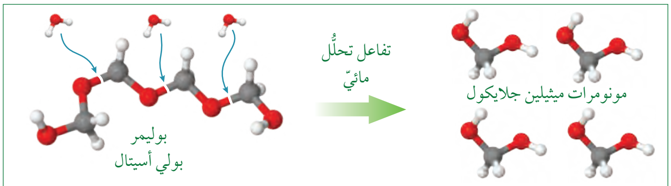
شكل 6-1 يفكّك التّحلّل المائيّ البوليمر عند الرّابطة بين المونومرات المتجاورة.
