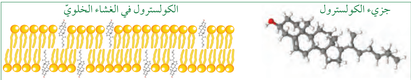
شكل 2-18 جزيء الكولسترول وموضعه في الغشاء الخلويّ.
