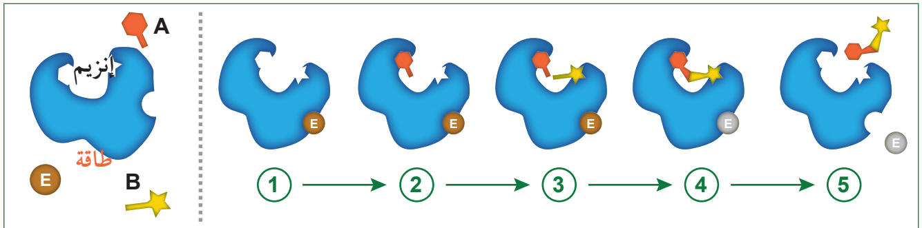
الشكل 3-12 نموذج القفل والمفتاح لتفاعل بناء ماص للطاقة.
