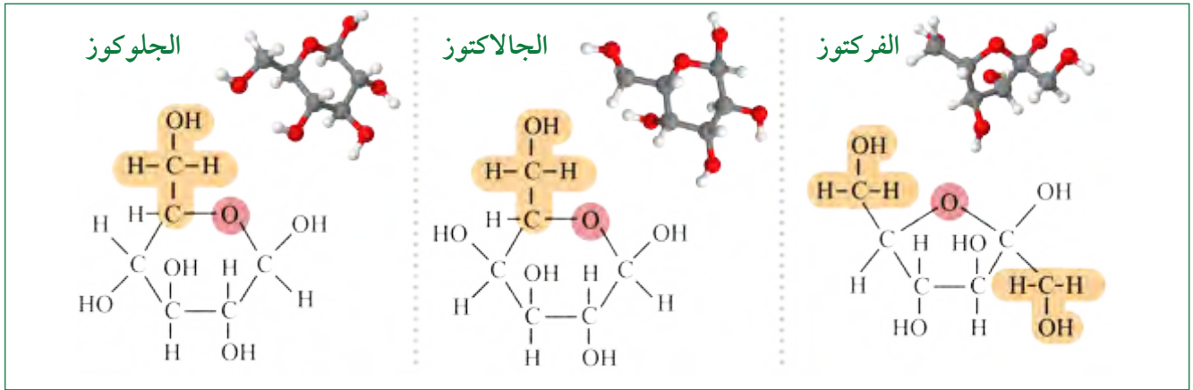
شكل 1-23 السكريات الأحادية سداسية الكربون الثلاثة الشائعة.
