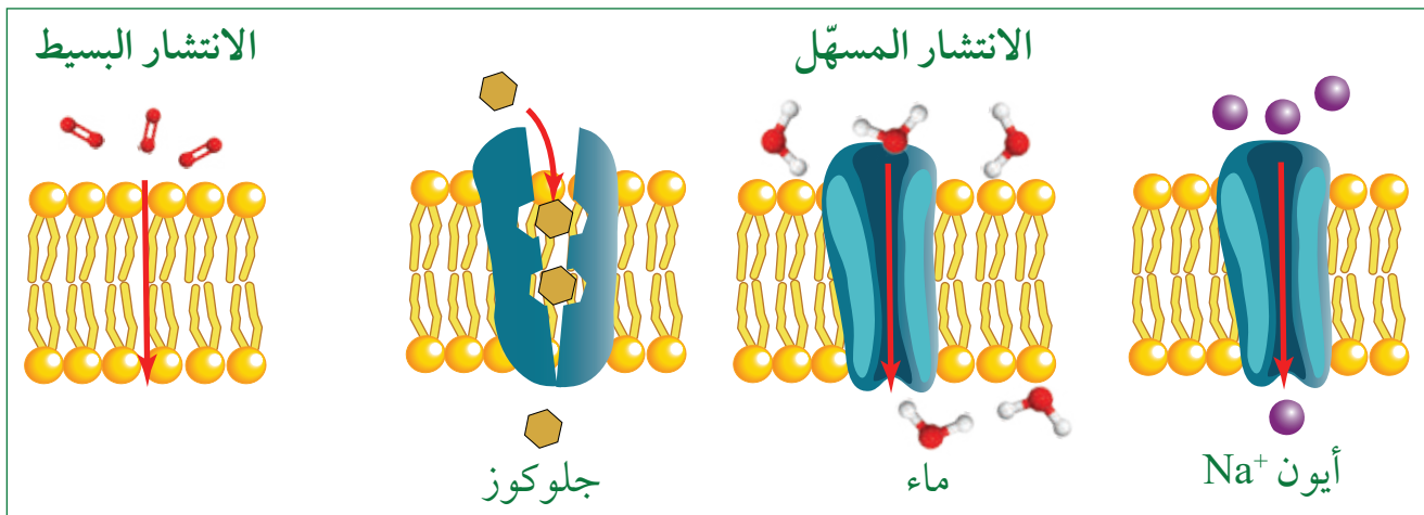
شكل 2-30 أربعة نماذج من النقل السلبي. البروتين الناقل يسهّل انتشار جزيئات الجلوكوز.
