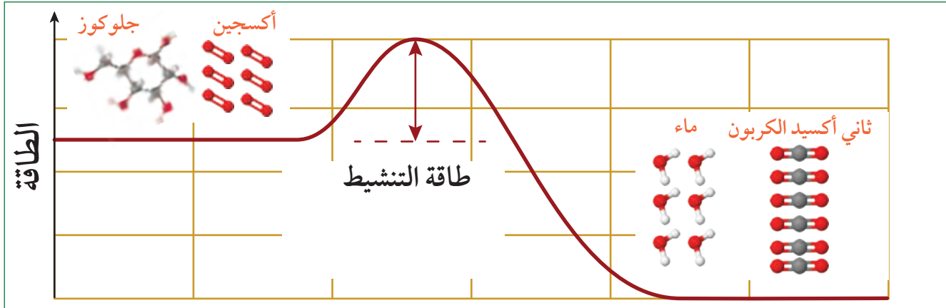
الشكل 3-6 طاقة التنشيط.
