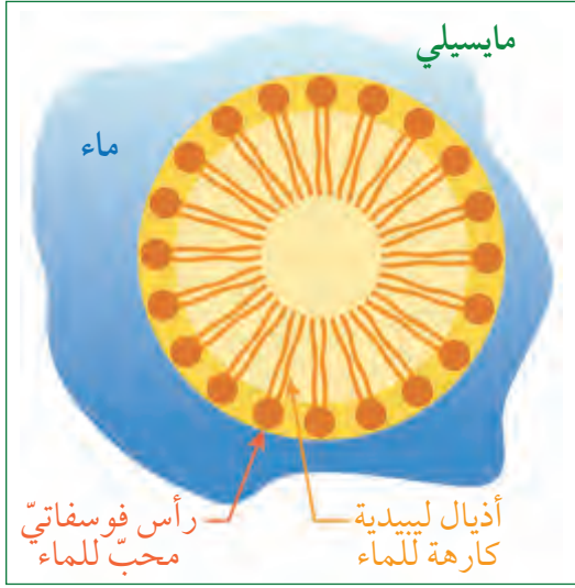
شكل 37-1 تشكّل الفسفوليبيدات مايسيليات في الماء.
