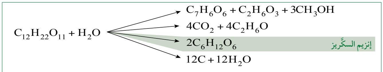
الشكل 9-3 يختار الإنزيم المحفز مسار التفاعل.
