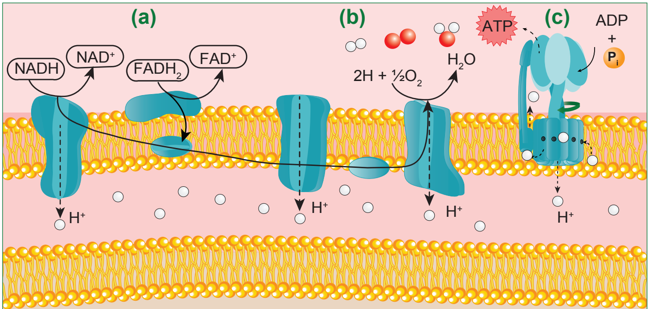
الشكل 24-4 سلسلة نقل الإلكترون مع مرافقات إنزيم ناقلة، (b) ذرّات الأكسجين تعمل بصفقتها مُستقبِلات إلكترونات كي تكوّن الماء، و (c) ATP سينثيز.
