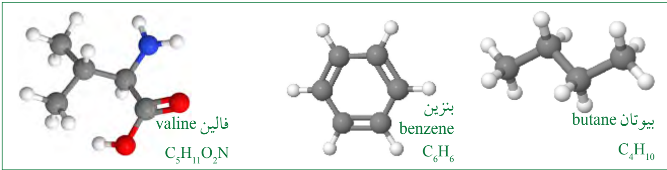
شكل 3-1 ثلاثة مركّبات كربون نموذجيّة.
