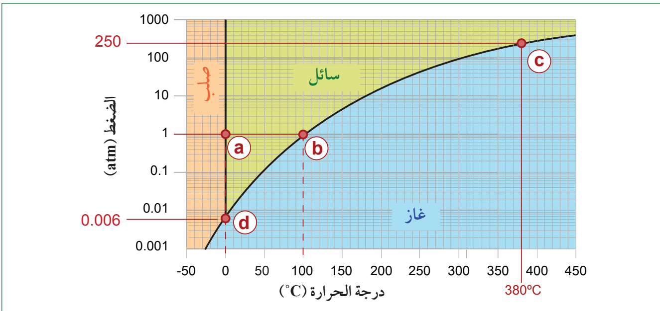
شكل 14-1 مخطط أطوار الماء.
