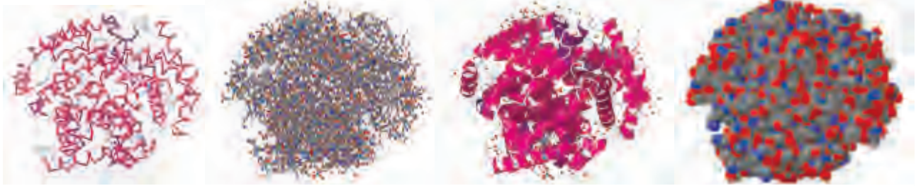
نمط ملء الفراغ نمط الشريط نمط الكرة والعصا نمط الهيكل الأساسي
