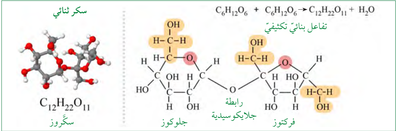
شكل 25-1 الرّابطة الجلايكوسيدية تربط بين حلقات السَّكَّر.
