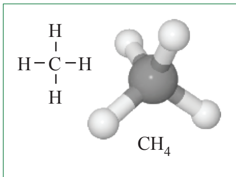
شكل 2-1 الميثان مركّب كربونيّ بسيط.
