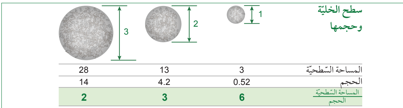
شكل 2-2 نسبة المساحة السطحيّة إلى الحجم لثلاثة أحجام خلويّة مختلفة.
