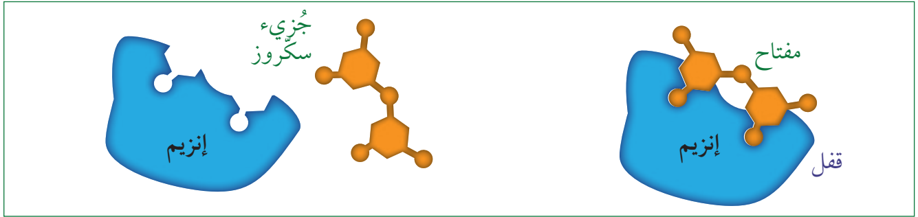
الشكل 3-11 نموذج القفل والمفتاح.
