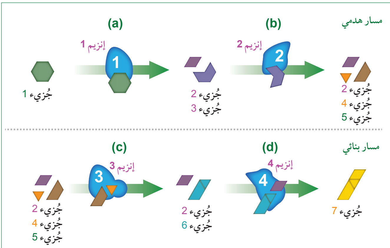
الشكل 3-18 نوعان من المسارات الكيميائية.
