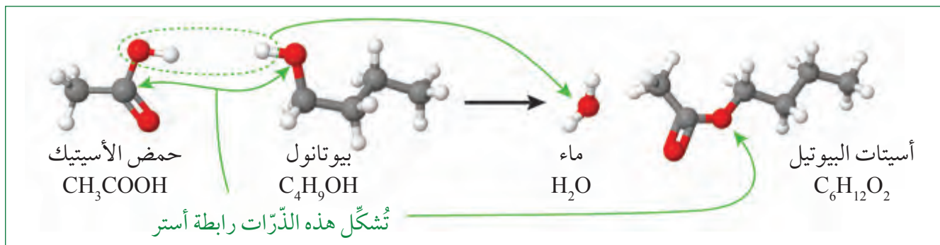
شكل 35-1 تشكّل رابطة استر في أسيتات البيوتيل في أثناء تفاعل تكثيفي.
