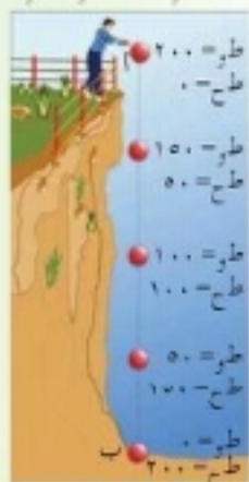
الشكل (٤-١٢): حفظ الطاقة الميكانيكية
