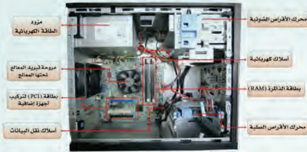
شكل (٥-١-٢): المكونات الداخلية لجهاز الحاسب
