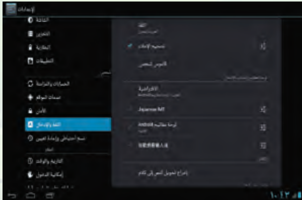
شكل (٣-٦-٥): شاشة إعدادات اللغة
