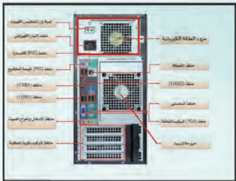
شكل (٢-١-٣): صندوق الحاسب من الخلف
