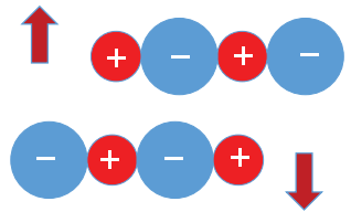
الشكل (32): تحطّم بلّورة المادّة الأيونية نتيجة تعرّضها للطّرق.
