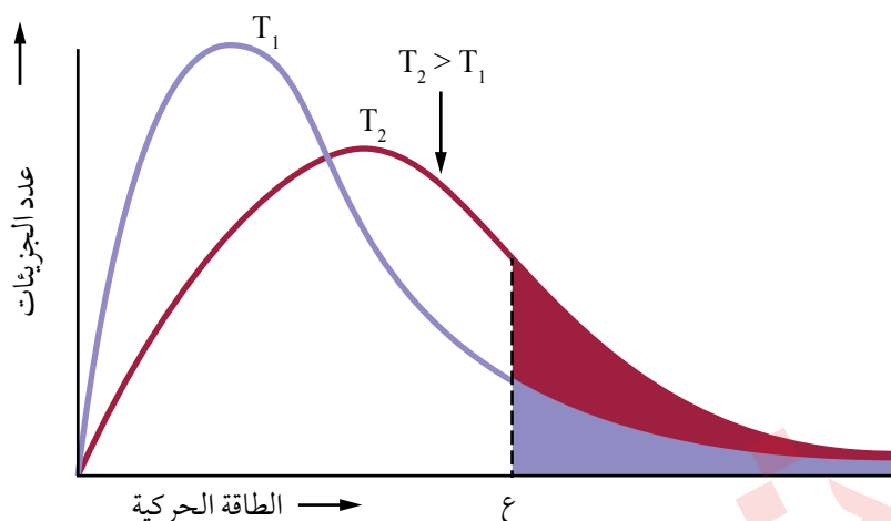
الشكل (17): منحني توزيع الطاقة الحركية للجزيئات عند درجتي حرارة T_1 و T_2 .
