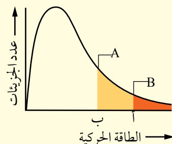
الجدول (2): طاقة التبخر المولية لعدد من السوائل عند درجة الغليان.
