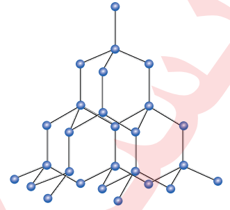
الشكل (26): رسم تخطيطي للماس.
