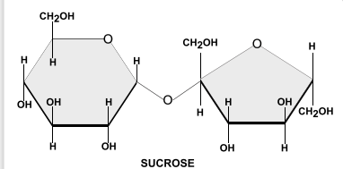
الشكل (6): جزيء سكر السكروز.
