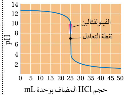
الشكل (7 / ب): منحنى معايرة قاعدة NaOH بالحمض HCl.
