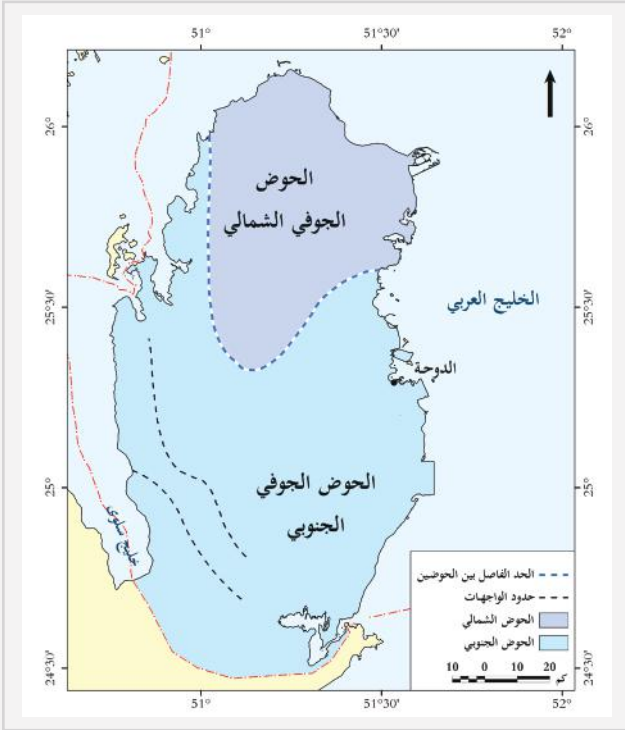
شكل (6) أحواض المياه الجوفية بدولة قطر
