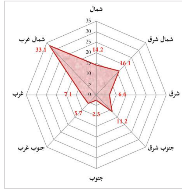
شكل (2) واردة الرياح بدولة قطر
