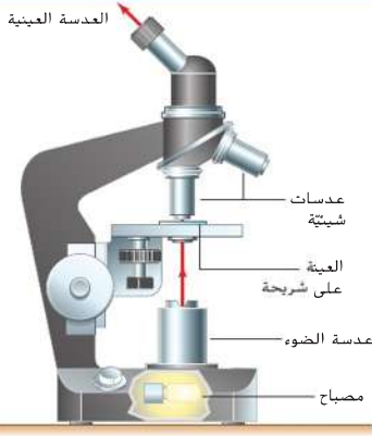
الشكل 26 تكوّن العدسة الشيئية والعدسة العينية في هذا المجهر المركب صورة معكوسة وأكبر مُعَارَنة بالجسم.
