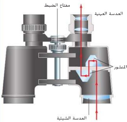
الشكل 27 يعمل المنظار بطريقة مماثلة للتلسكوب الكاسر.
