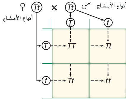
■ الشكل 12 تُعد قدرة الفرد على ثني لسانه صفة سائدة. يعد مربع بانيت ملخصاً مرئياً لاحتمالات ارتباط الأليلات الخاصة بصفة ثني اللسان.
