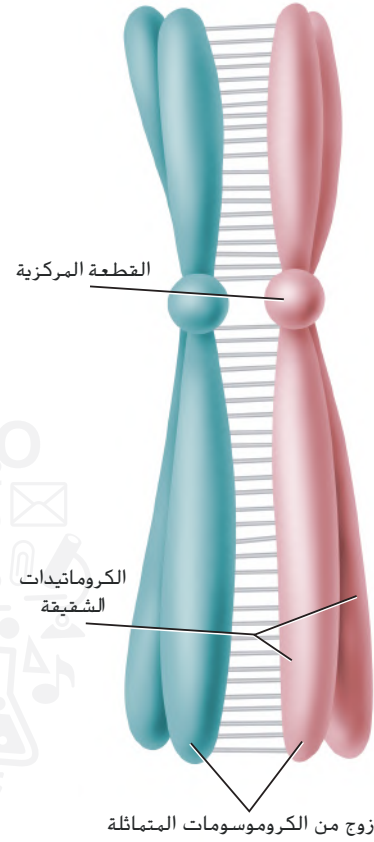
■ الشكل 3 تتلاصق الكروموسومات المتماثلة معًا أثناء عملية التشابك في الطور التمهيدي الأول.
