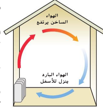
الشكل 5 تحدث تيارات الحمل عندما يتصاعد الهواء الأكثر دفئًا والأقل كثافة إلى أعلى ويهبط الهواء الأكثر برودة وكثافة.
