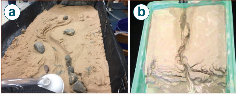
الشكل 2-36 يبين الحوض المائل التعرية.
