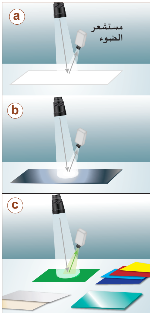
الشكل 3-14 إعداد المختبر.
