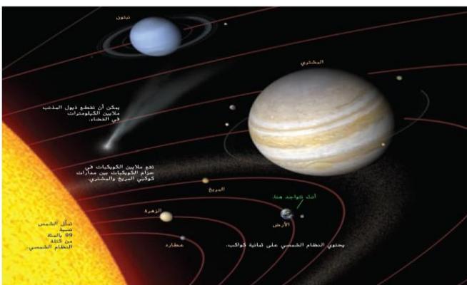
الشكل 11 يشرح النظام الشمسي الشمس والكواكب والعديد من الأجسام الأخرى.
