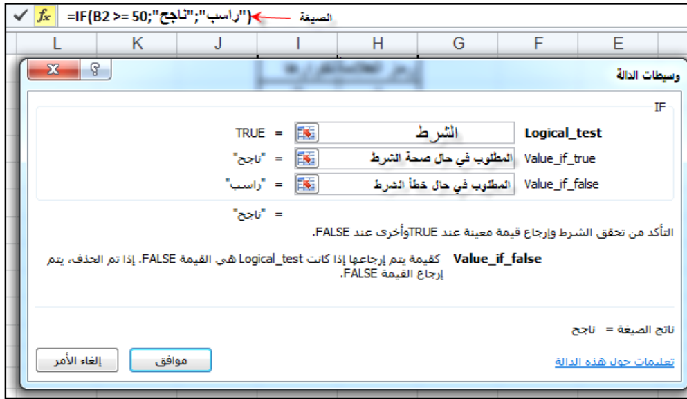
الشكل (٤-٦٠): صندوق الحوار وسيطات الدالة
