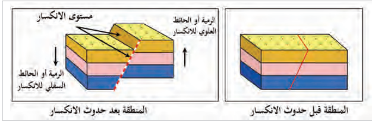
شكل (1) مثال لمنطقة قبل حدوث انكسار وبعد حدوثه
