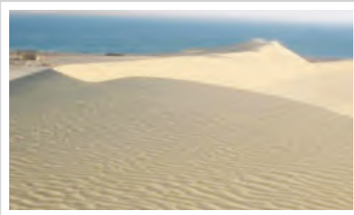
كثيب طولي (سيفي)
