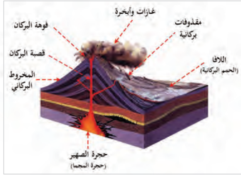
شكل (2) أجزاء البركان
