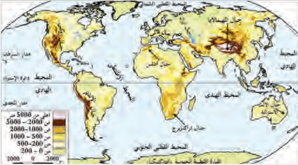
شكل (4) توزيع الجبال الالتوائية في العالم
