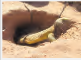
التجوية بفعل الحيوانات
