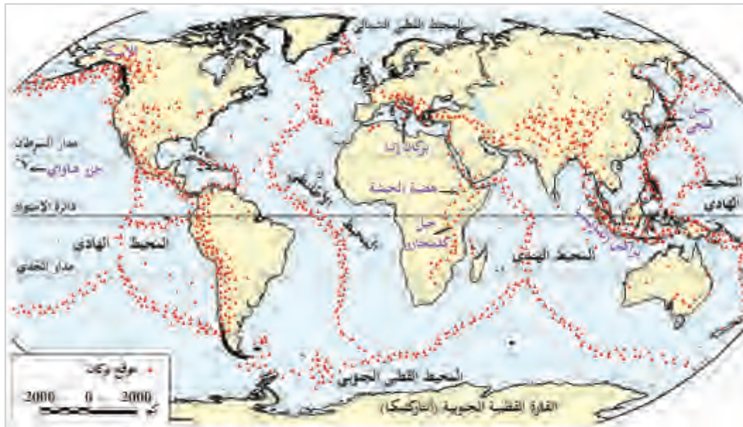
شكل (3) التوزيع الجغرافي للبراكين
