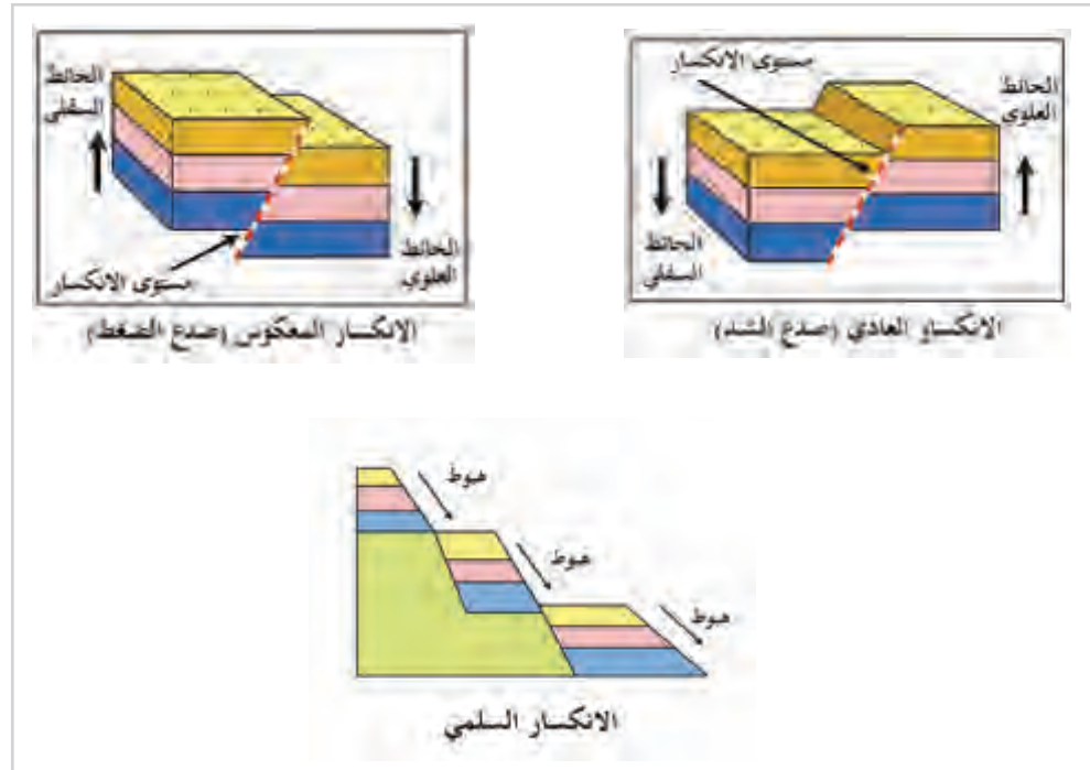
شكل (2) أنواع الانكسارات
