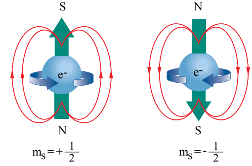
الشكل (12): الدوران المغزلي للإلكترون.
