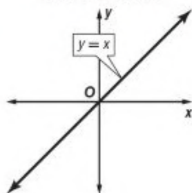
Linear Functions
