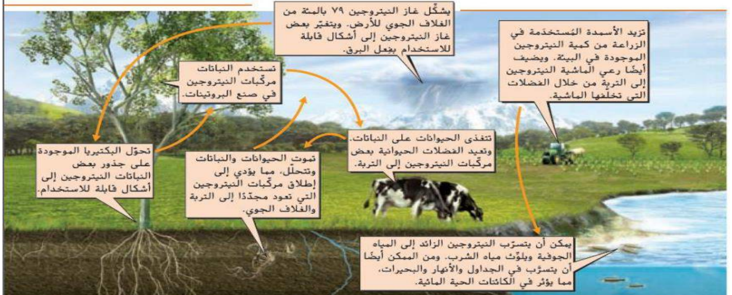
الشكل 5 يمكن أن يؤدي الممارسات الزراعية إلى زيادة كمية النيتروجين الذي يمرّ خلال دورته عبر الأنظمة البيئية.
