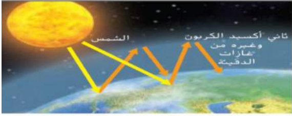
الشكل 19 تلتصق غازات الدفيئة الطاقة الحرارية من الشمس ثم تُعيد إشعاعها وتؤدي إلى تدفئة سطح الأرض.
