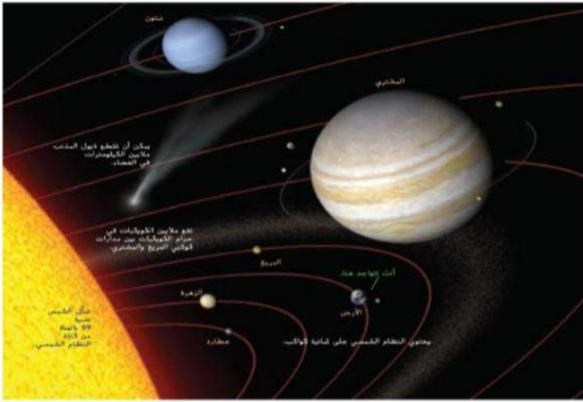
الشكل 11 يشرح النظام الشمسي والكواكب والمذنبات من الأجسام الأخرى.
