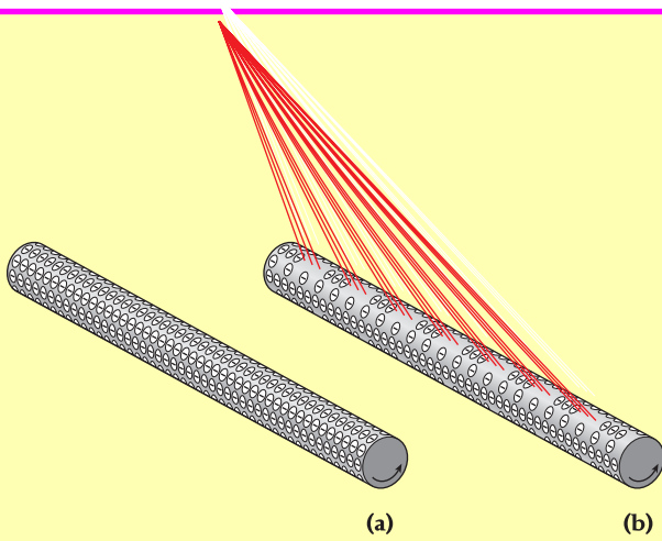
الشكل 1.22 (a) الأسطوانة المشحونة بالكامل في طابعة الليزر. (b) أسطوانة يتم تسجيل سطر واحد من البيانات عليها بواسطة ضوء الليزر. حيث تتعادل الشحنة السالبة عند أي نقطة يسقط عليها ضوء الليزر، فتجذب النقاط مفرغة الشحنة مسحوق الحبر الذي ينتج صورة على الورقة.
