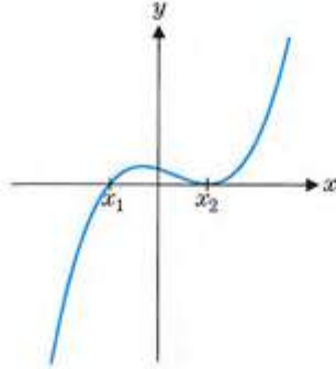
الشكل 1.23b صفران اثنان
