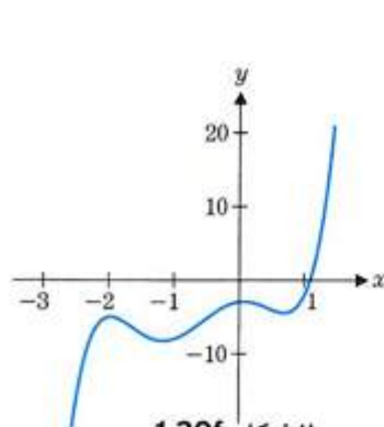
الشكل 1.20f f(x) = 2x^5 + 6x^4 - 8x^2 + x - 3
