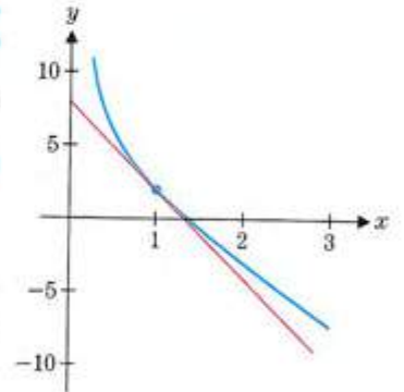
الشكل 3.22 y = f(x) والمماس عند x = 1
