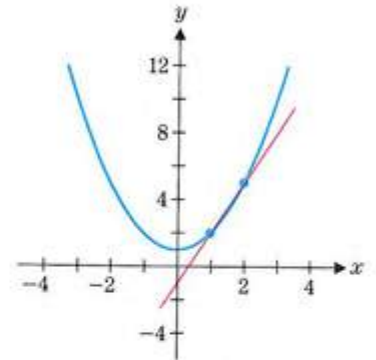
الشكل 3.4b القاطع الذي يربط بين (1, 2) و (2, 5)
