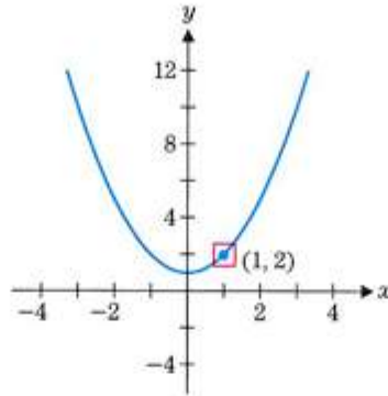
الشكل 3.2 y = x^2 + 1
