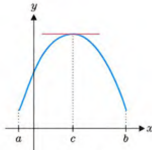
الشكل 3.48a تمثيل بياني بشكل متزايد في البداية
