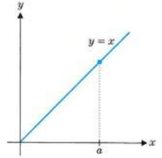
الشكل 3.21 المماس مع y = x
