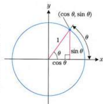
الشكل 1.38 تعريف \sin \theta و \cos \theta : \cos \theta = x و \sin \theta = y
