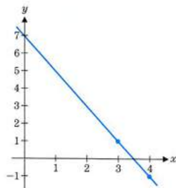
الشكل 1.14 y = -2(x - 3) + 1
