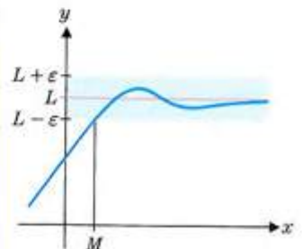
الشكل 4.55 \lim_{x \rightarrow \infty} f(x) = L
