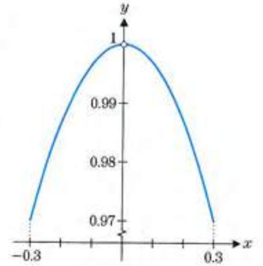
الشكل 2.17 y = x \cot x
