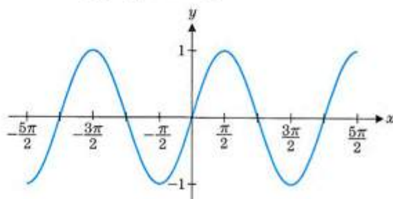
الشكل 1.39a y = \sin x
