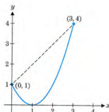
الشكل 2.5a y = (x-1)^2
