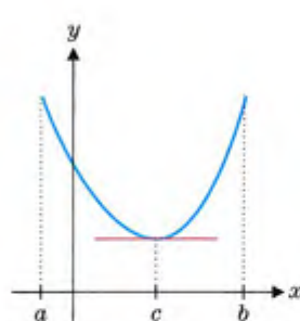
الشكل 3.48b تمثيل بياني بشكل متناقص في البداية
