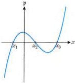
الشكل 1.23c ثلاثة أصفار
