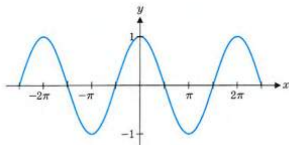
الشكل 1.39b y = \cos x
