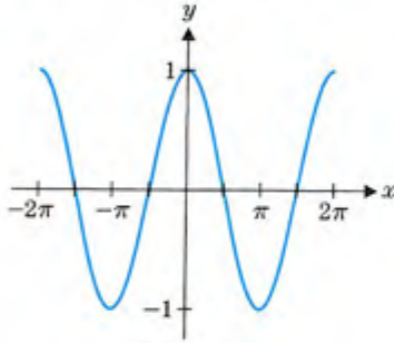
الشكل 5.26b مشتقة f(x) = \sin x
