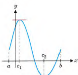
الشكل 3.48c تمثيل بياني بمماسين أفقيين
