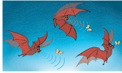
خفافيش تستخدم الموجات فوق الصوتية لمطاردة فريستها.
