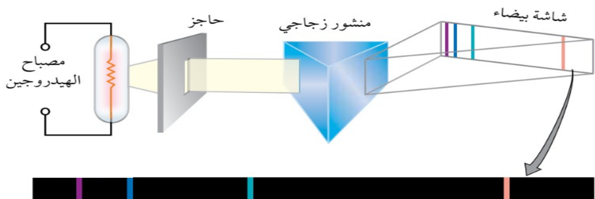
الطيف الخطي (المنفصل) الناتج من تحليل ضوء مصباح الهيدروجين.
