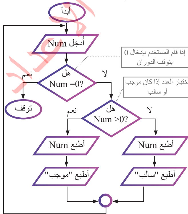
الشكل (2-11): مُخطَّط سَير العمليات لإدخال مجموعة أعداد، وتصنيفها إلى موجبة وسالبة
